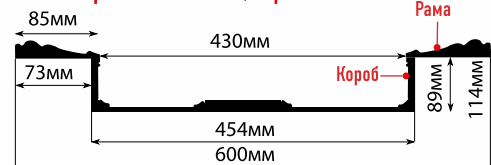
KS61A-58 рама: 600x600x25, короб: 454x454x89
