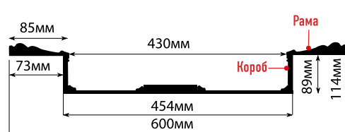
KS61A-19D рама: 600x600x25, короб: 454x454x89
