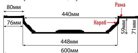
KS61-56 рама: 600x600x12, короб: 448x448x59
