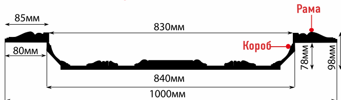
КР100-59 (1000х1000х98) рама: 1000х1000х20 короб: 848х848х78
