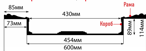
KS61A-18D рама: 600x600x25, короб: 454x454x89
